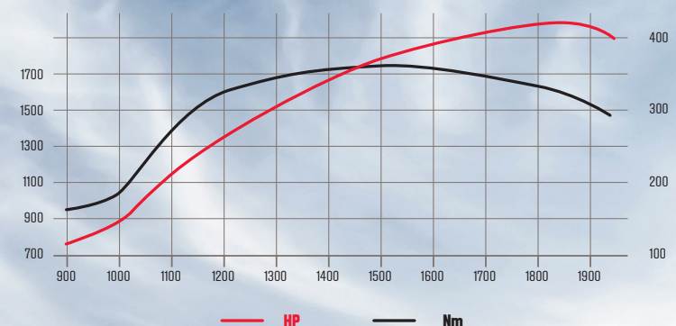
ВЪРТАЩ МОМЕНТ В NM, S394 И S416
